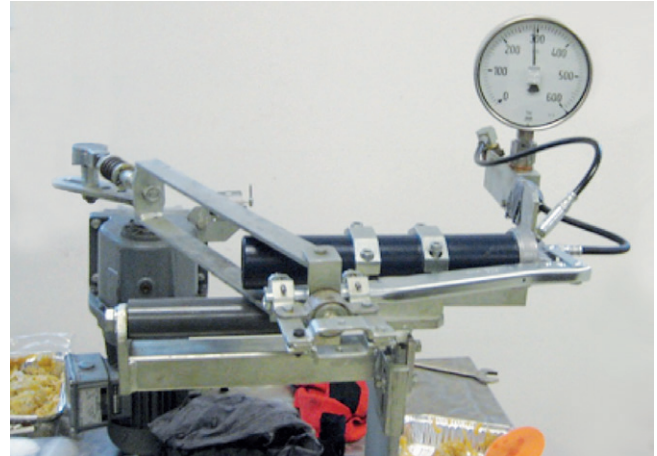
Bild 2: Prüfstandstest nach DIN 1283
